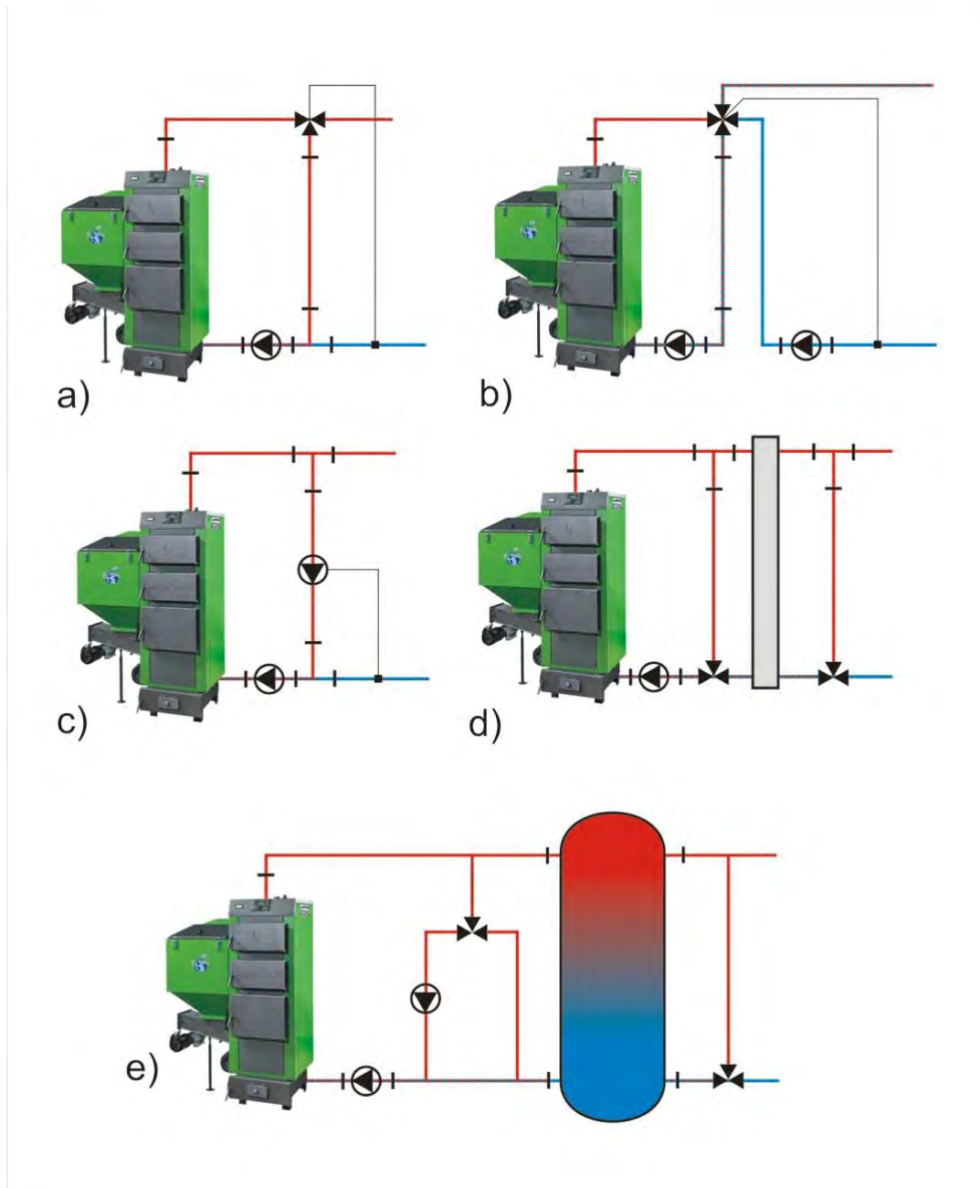
Рис 5. Рекомендуемые схемы соединения котла MULTI с системой отопления: а) с трехходовым клапаном; б) с четырехходовым клапаном; в) с циркуляционным насосом; д) с гидравлической муфтой; е) с буферной ёмкостью
