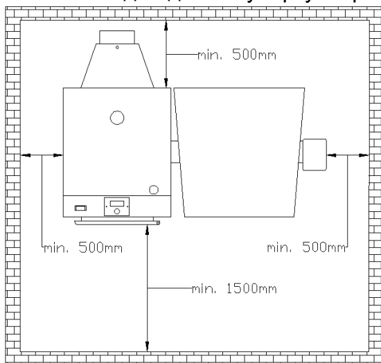
Рис 3. Установка котла в котельной
