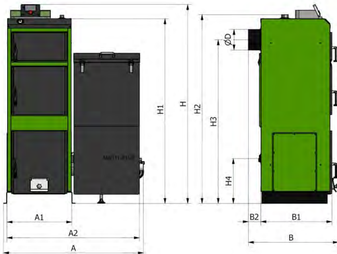
Рис 2. Размеры котла MULTI plus
