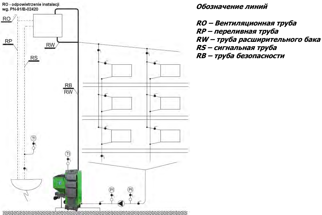
Рис. 4. Пример схемы защиты водяного отопления оснащенного одним котлом, насос установлен на возврате ( PN-91/B-02413)
