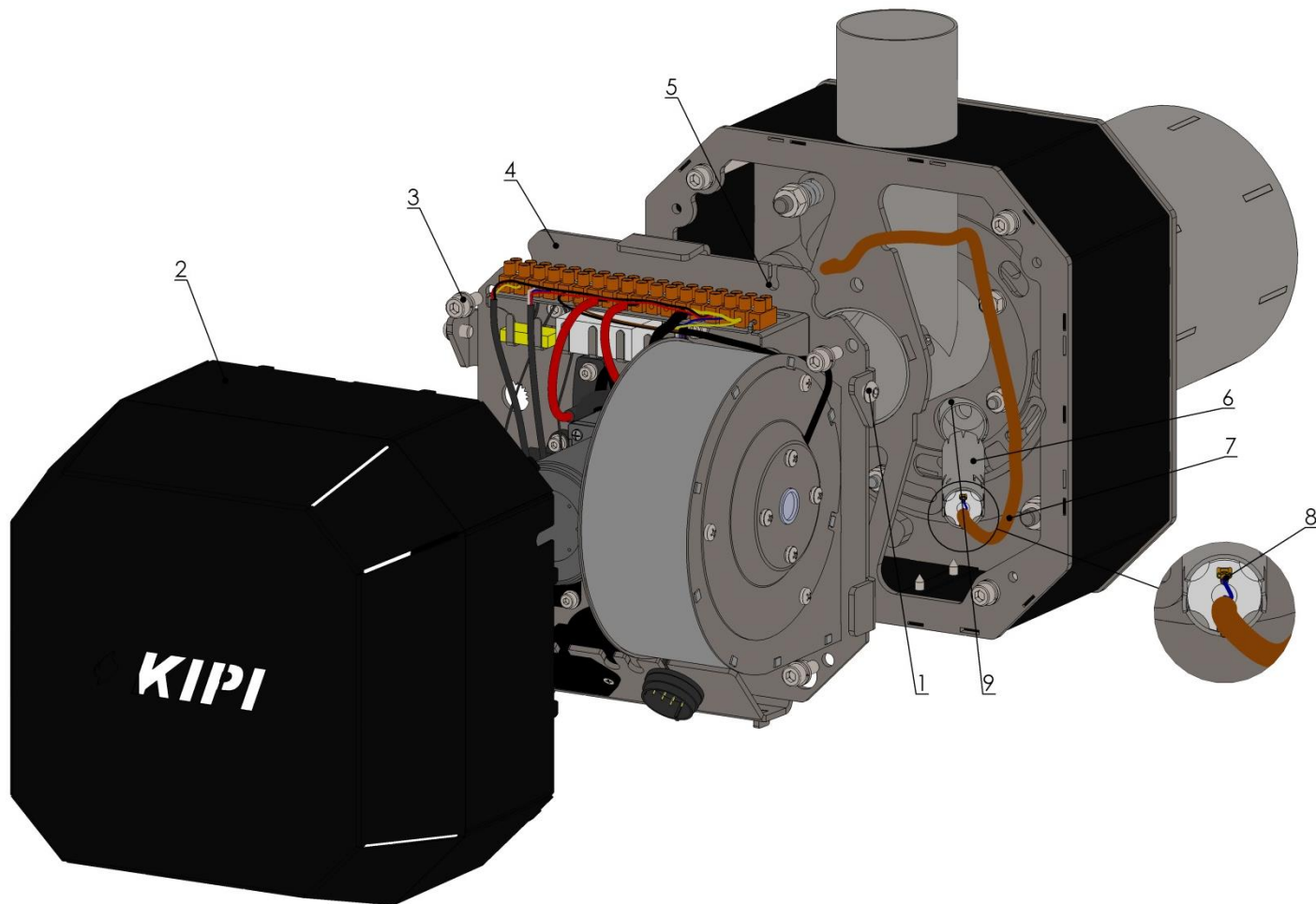
Рис. 13. Замена воспламенитель.
