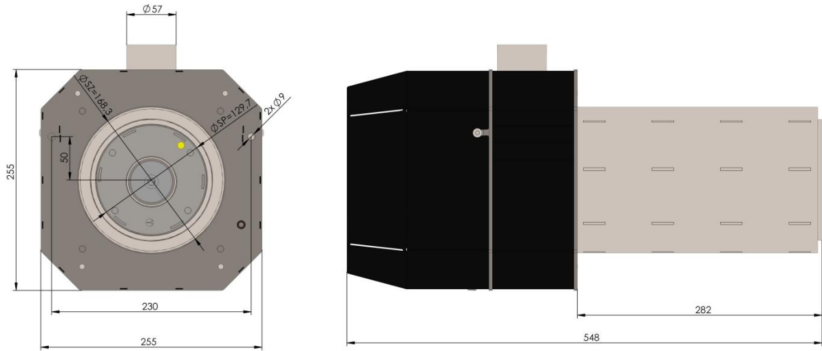
Рис. 24. Вид горелки 10-50kW.
