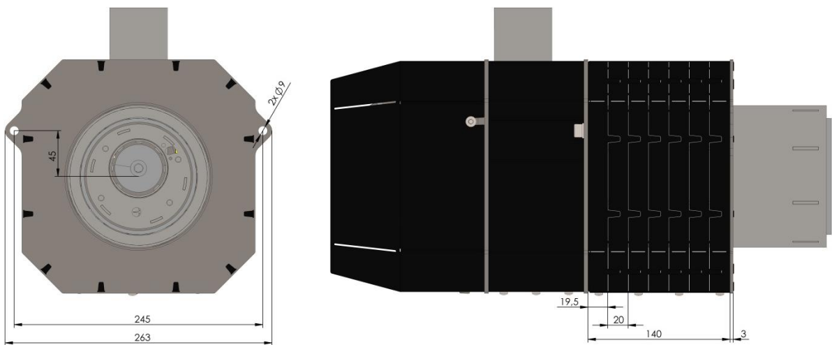
Рис. 22. Вид горелки 8-36 kW.
