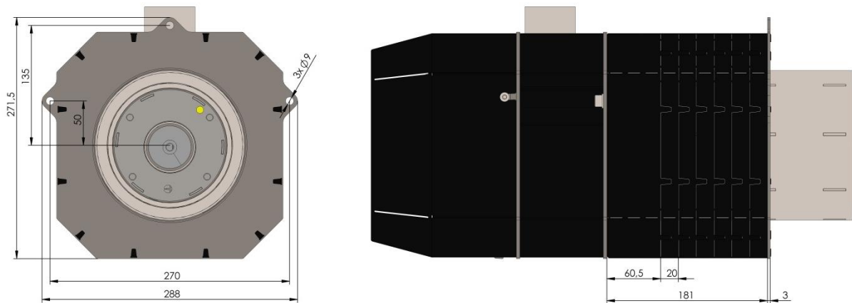
Рис. 25. Вид горелки 10-50 кВт тепловой изоляции рубашкой и монтажной пластиной.
