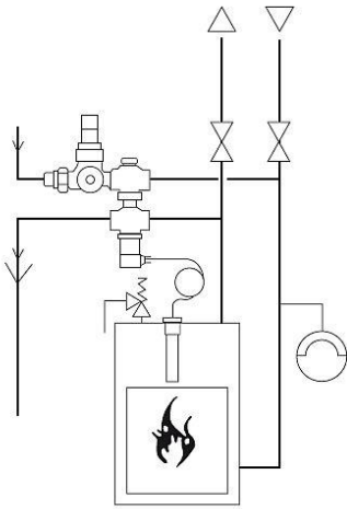
Рис. 6. Пример тепловой защиты
